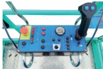
Einfacher und intuitiver Bedienpult, den man zum Laden / Entladen der Maschine aus der Plattform schnell runter nehmen kann
