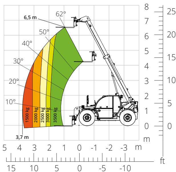
Diagramma di carico su pneumatici
